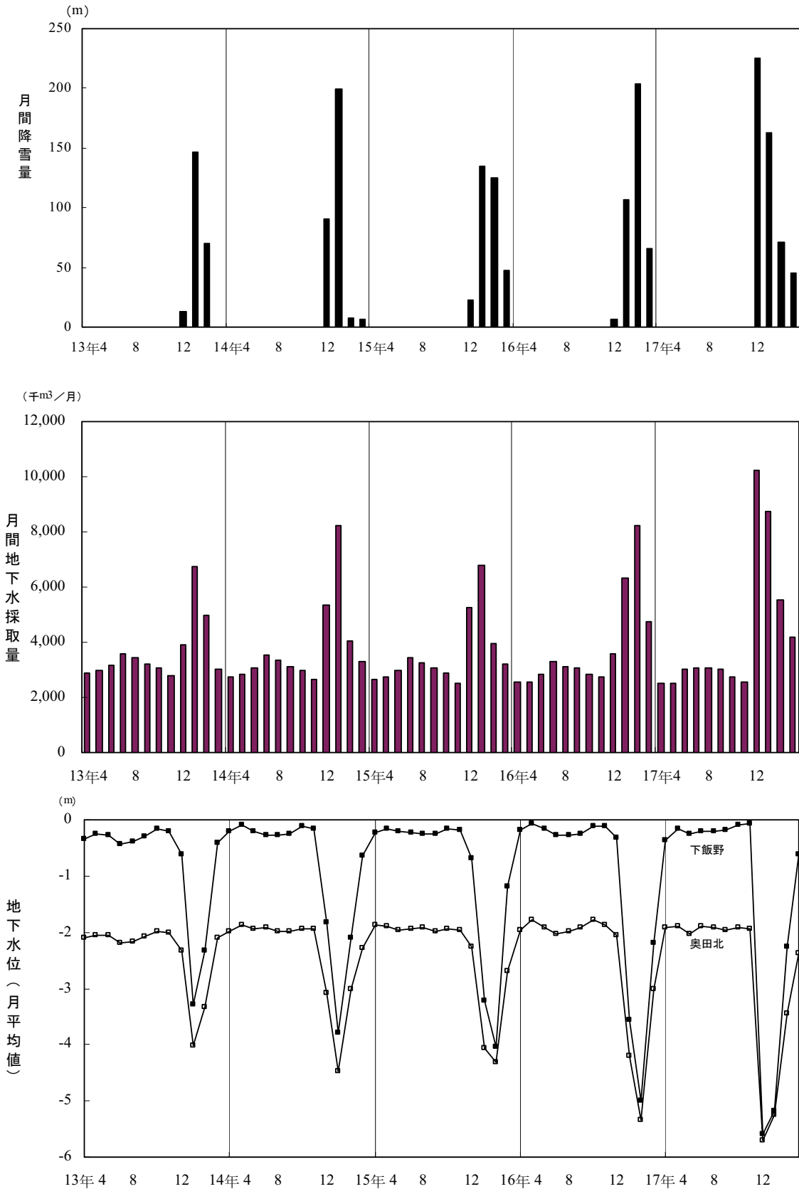
図 10-2 降雪量、地下水採取量及び地下水位の関係
