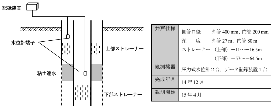
図7 中田地下水観測井概要図
