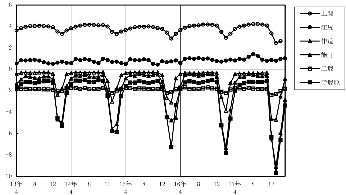
図9-1 地下水位 (月平均値) の経年推移
