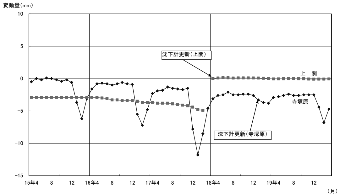
図12 地盤変動量
