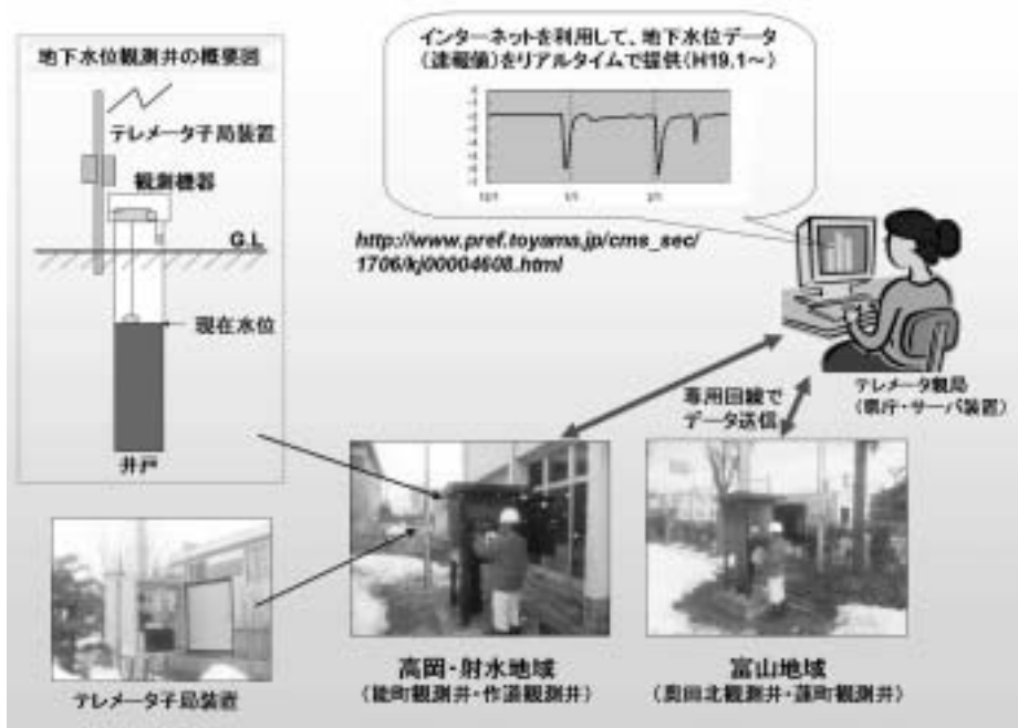
図7 テレメータシステム概要図
