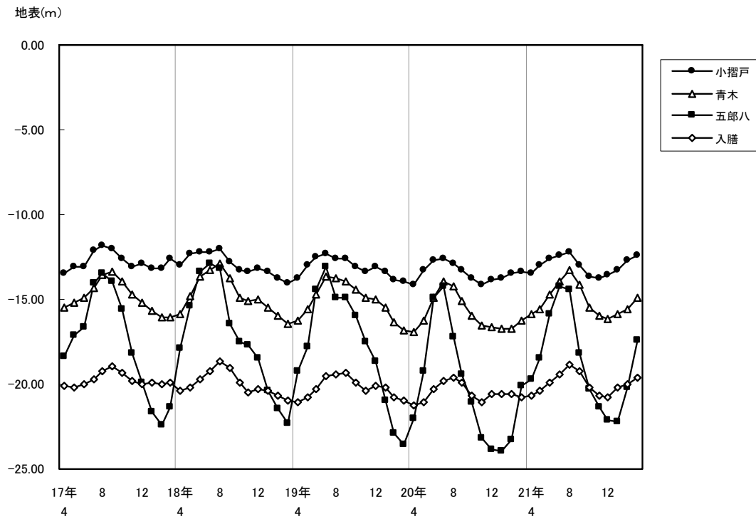
図 10-4 地下水位（月平均値）の経年推移
