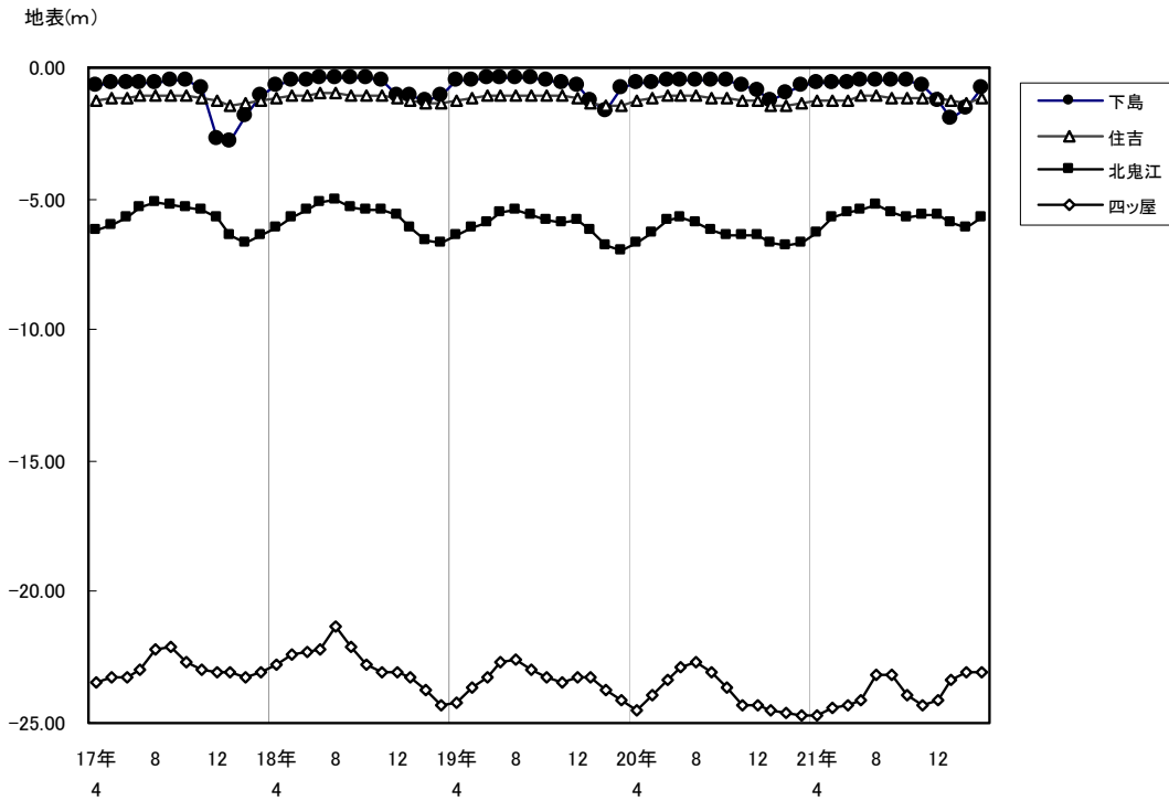
図 10-3 地下水位（月平均値）の経年推移
