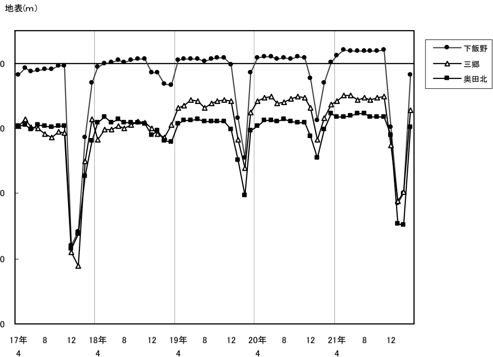
図 10-2 地下水位（月平均値）の経年推移
