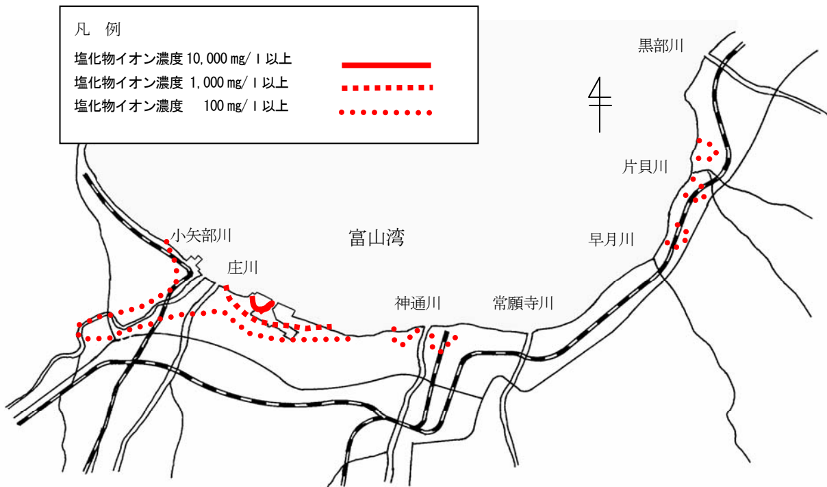
図 12 塩化物イオン濃度分布 (21 年度)
