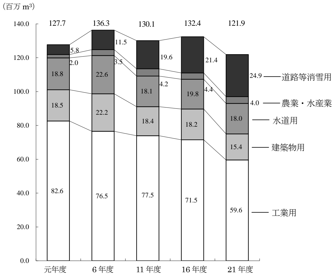
図4 用途別採取量の経年変化
