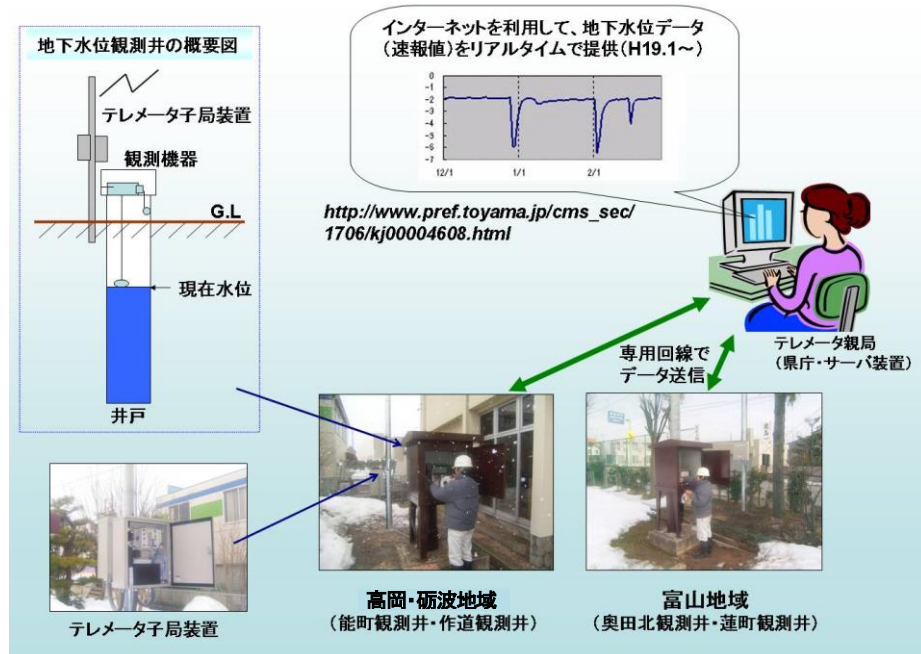
図8 テレメータシステム概要図
