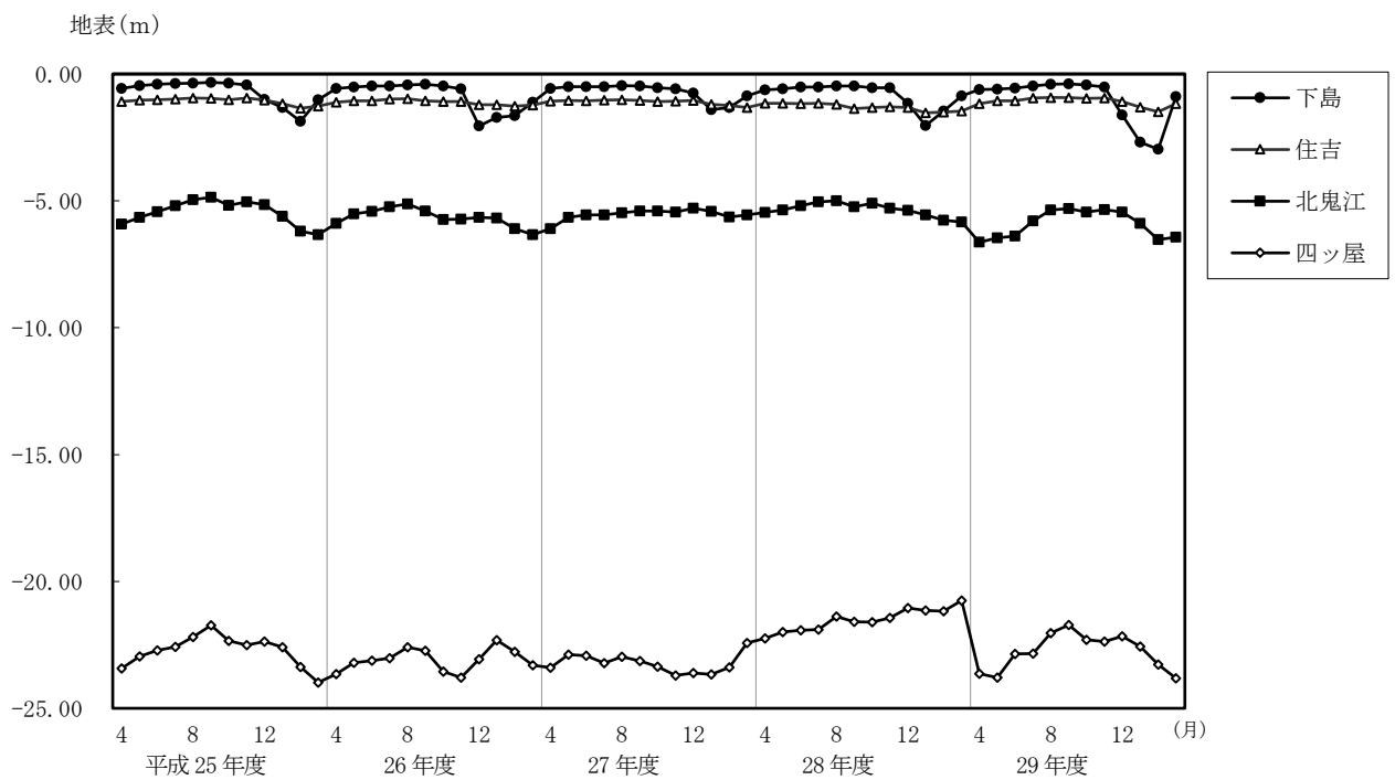
図 10-3 地下水位 (月平均値) の推移
