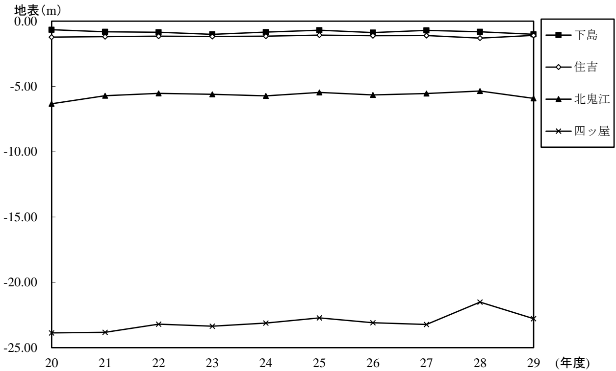
図9-2 地下水位（年平均値）の推移
