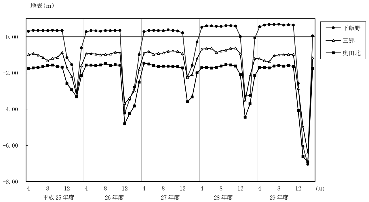
図 10-2 地下水位 (月平均値) の推移
