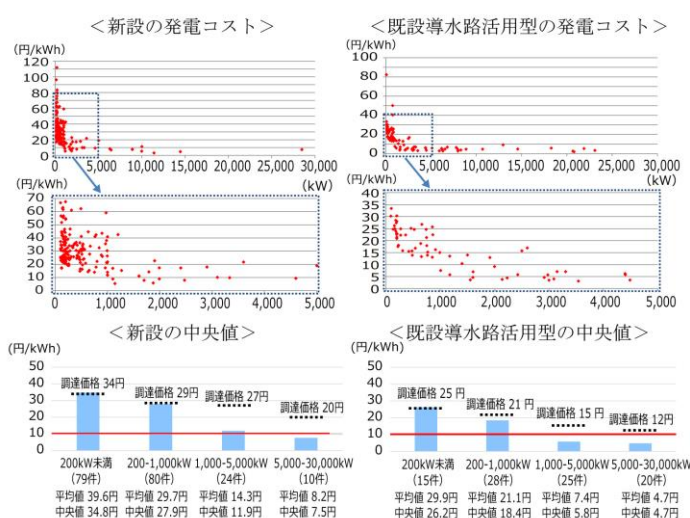
図 2-15 中小水力発電の出力と発電コストの関係
