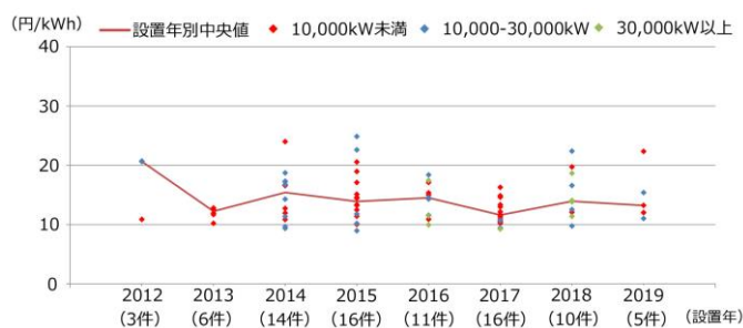
図2-12 陸上風力発電の発電コストの推移
