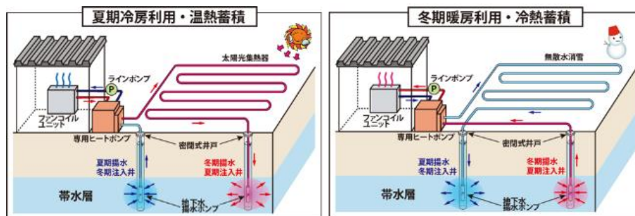
図 2-18 帯水層蓄熱システム
