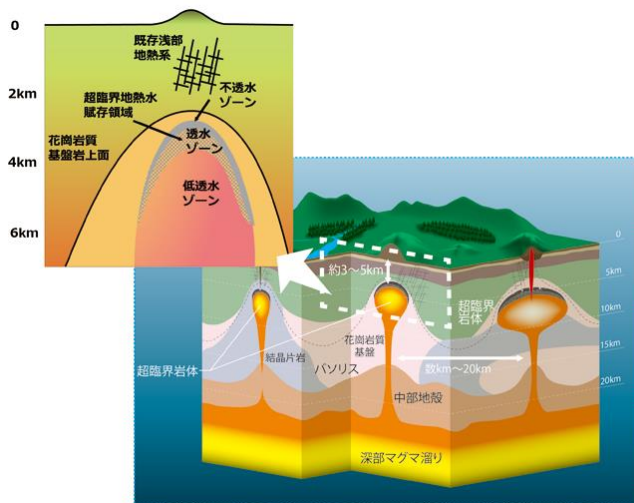
図 2-14 超臨海地熱発電に利用する地熱のイメージ
