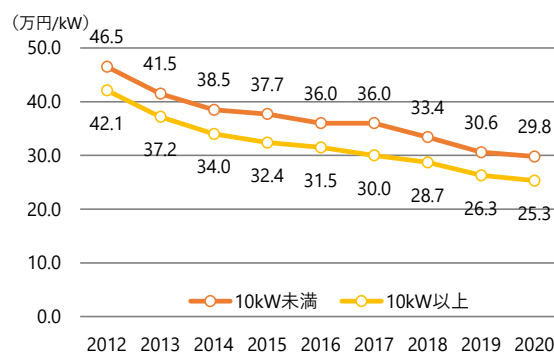
図2-10 太陽光発電のシステム費用の推移
